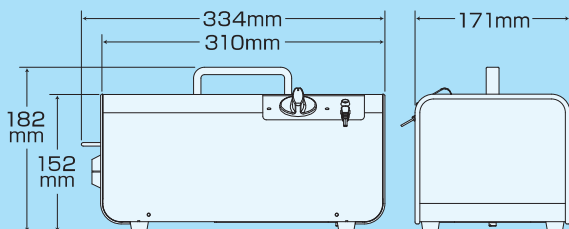
寸法図
