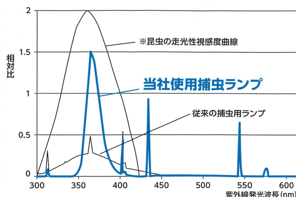
■当社使用捕虫ランプ紫外線出力と、イエバエの紫外線感度の 相関イメージ図および従来ランプとの比較
